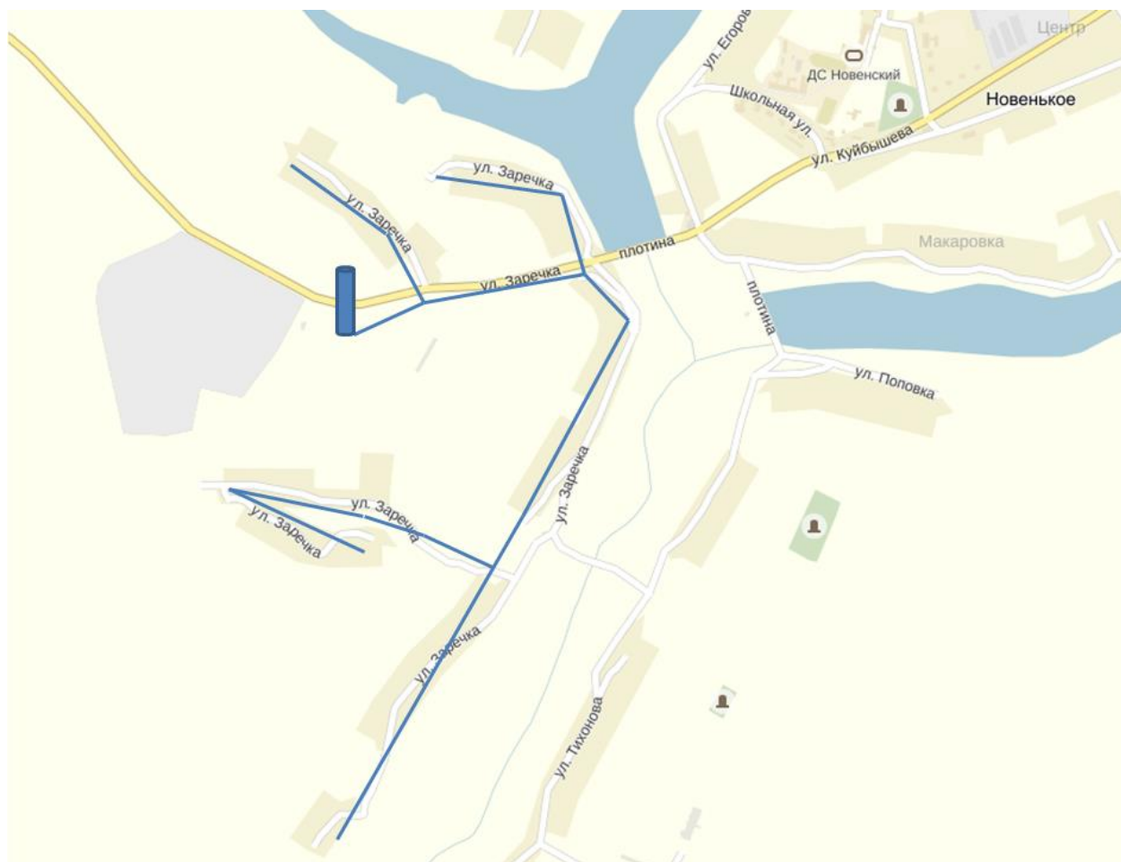
Рисунок 3. Схема водопроводной сети ул. Заречка
