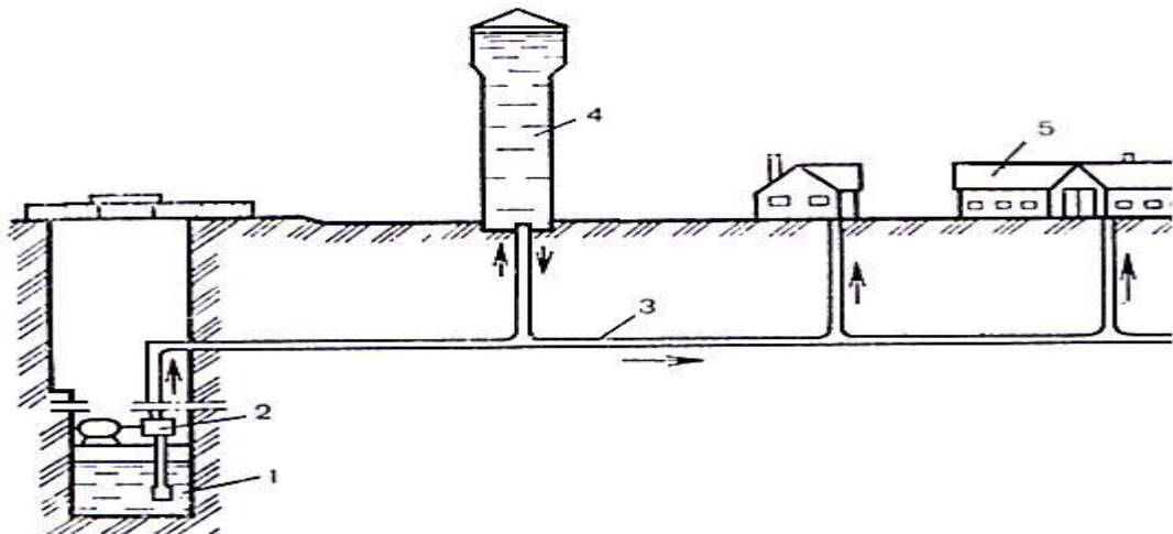
Рисунок 1. Структура системы водоснабжения.
