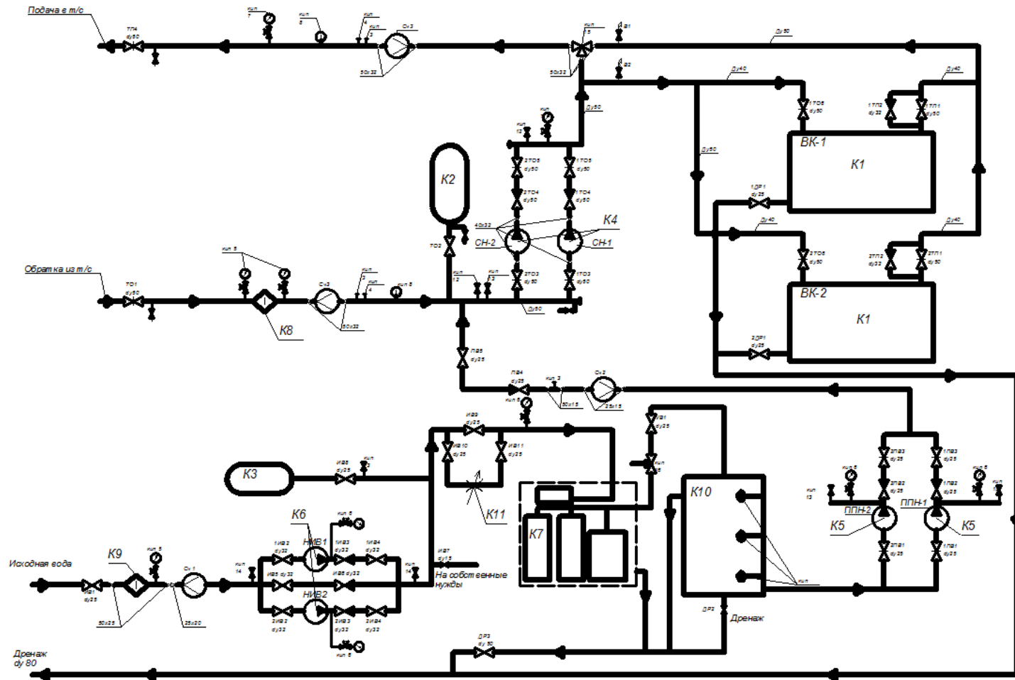
Рисунок 3.1 Схема отпуски тепловой энергии ТКУ-0,2 с. Богатое
