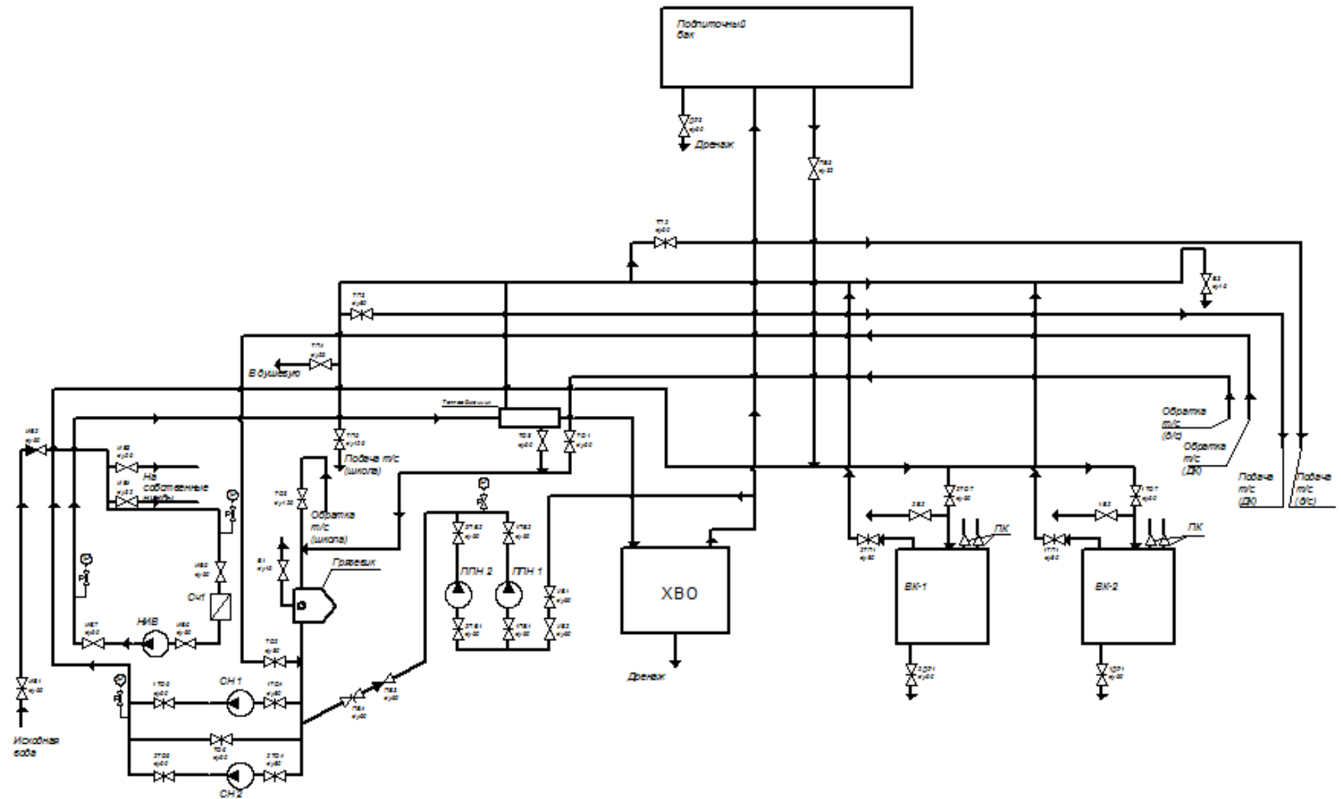
Рисунок 3. Схема отпуска тепловой энергии котельной с. Курасовка
