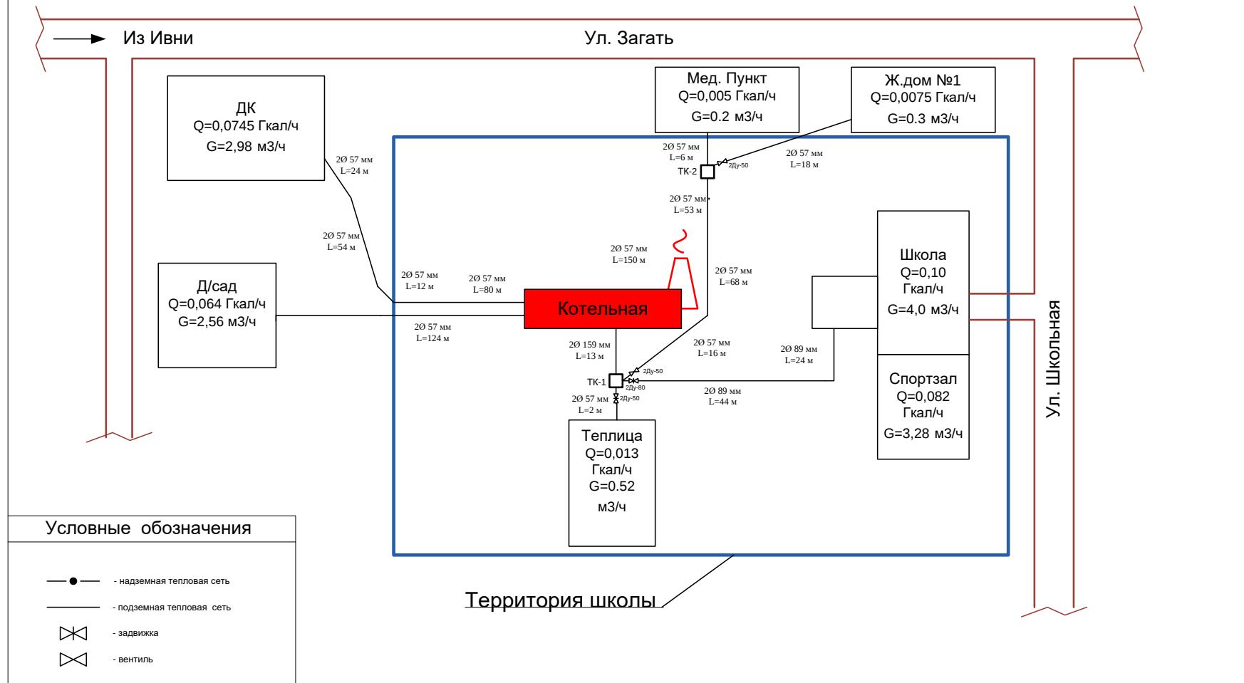
Рисунок 2. Схема тепловых сетей котельной с.Курасовка
